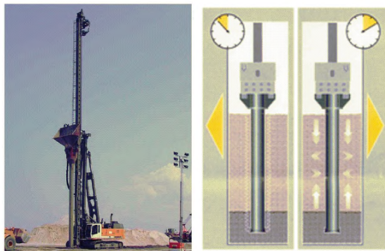
а - опускание трубы-лидера до прочного грунта; б - засыпка песка в геооболочку; в - выемка трубы-лидера с виброуплотнением песка в свае
